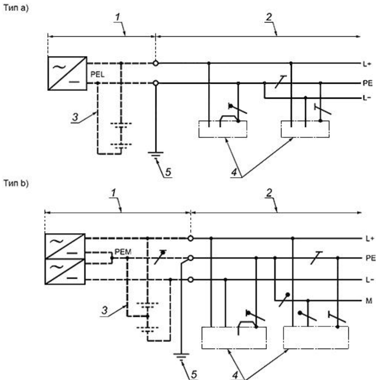
Рисунок 31К - Системы TN-C-S постоянного тока
