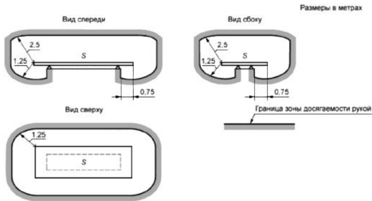
Рисунок 20.1 - Зона досягаемости рукой
