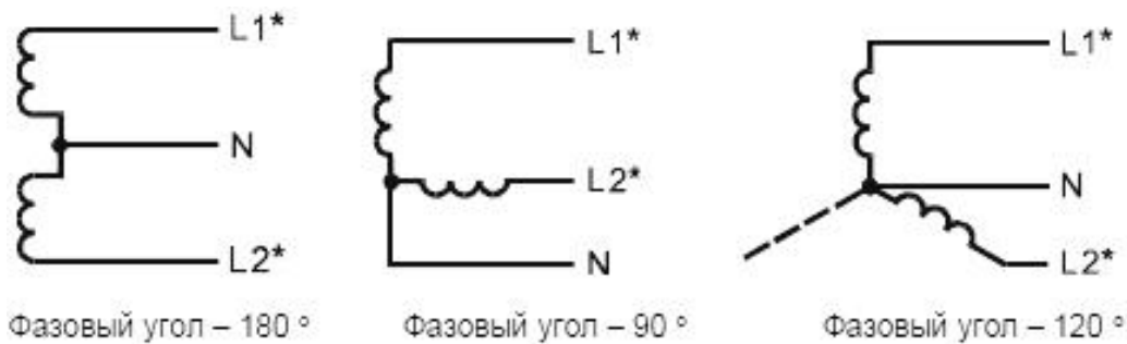
Рисунок 3 - Двухфазные трехпроводные электрические цепи
