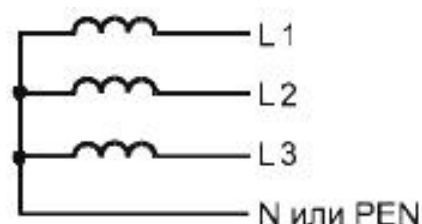
Рисунок 5 - Трехфазная четырехпроводная электрическая цепь
