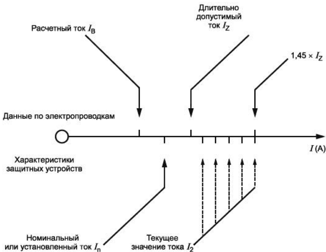
Рисунок В.1 - Иллюстрация условий 1 и 2 из 433.1
