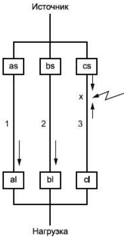
Рисунок А.3 - Электрический ток в начале отказа
